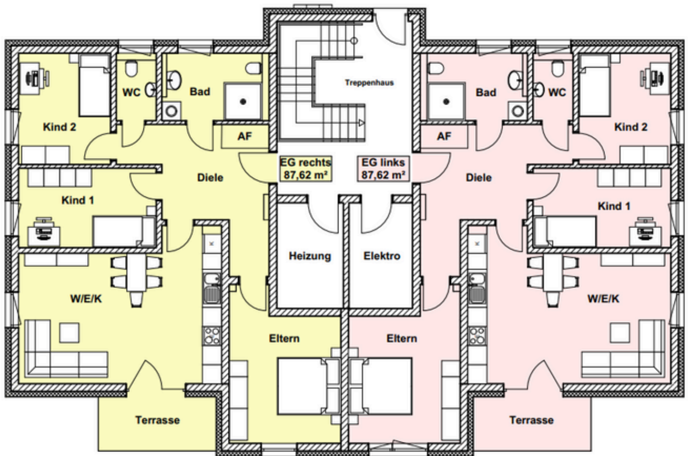
Erdgeschoss
